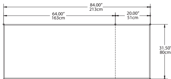
Plan View F2984VDR, F2984VDR-CE
