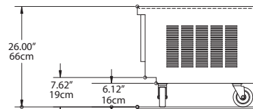
Right End View F2984VDR, F2984VDR-CE
